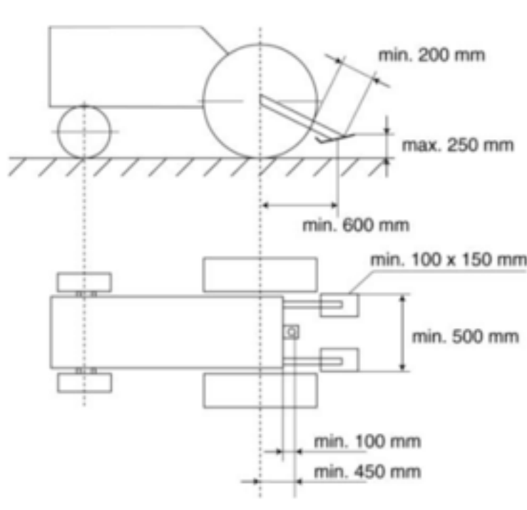
Figuur 1 : Steigerbegrenzer
